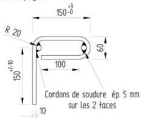
Figure 21 - EXEMPLES de BOUCLES de LEVAGE et POSITIONS des BOUCLES de LEVAGE
