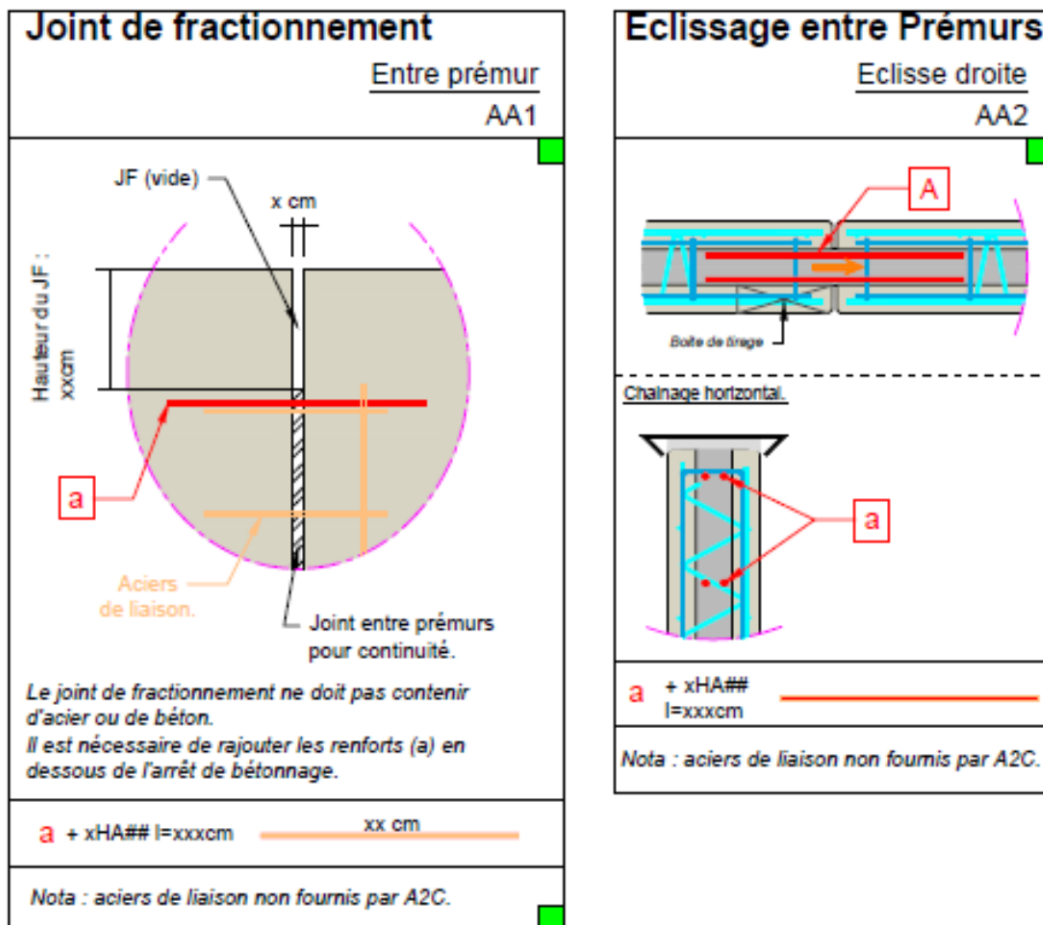
Figure 18 – ACROTÈRES - 1
