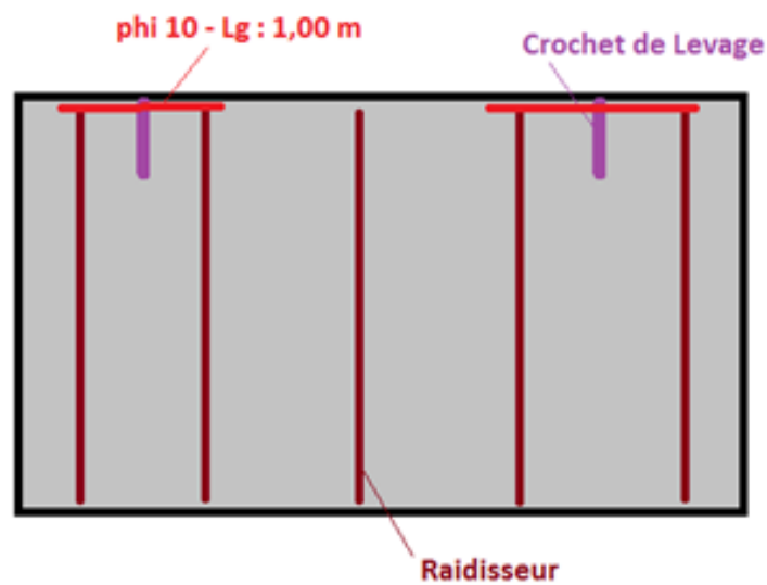
Figure 25 - Position des aciers de renfort au droit des boucles de levage : Diamètre 10 mm, Longueur 1,0 m
