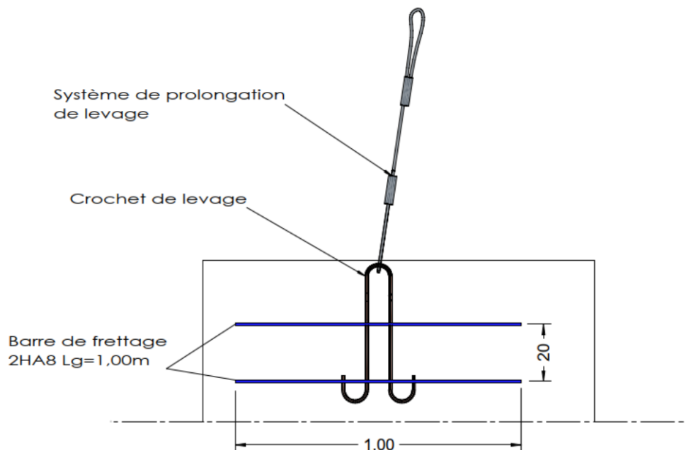
Figure 29 – MISE EN OEUVRE des INSERTS de LEVAGE Crochet A2C dans la peau des PREMURS A2C
