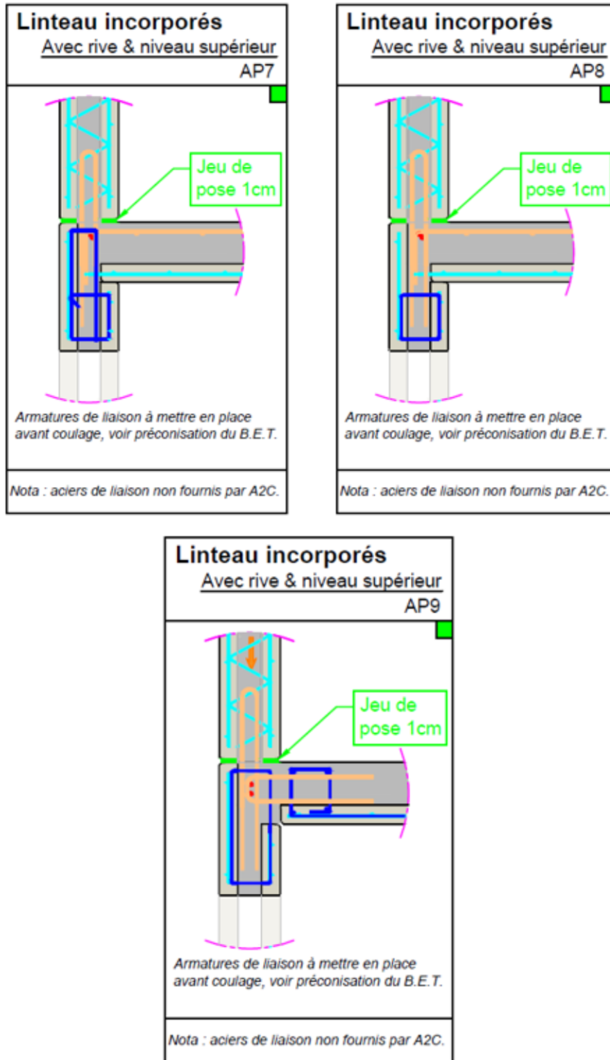
Figure 7 - LIAISONS ARTICULEES - 1
