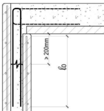
Figure 1 - Reprise de bétonnage dans le cas d'une dalle
