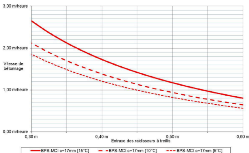
Figure 2 - Vitesse de bétonnage pour les BPS en fonction de la température et de l'entraxe des raidisseurs (pour un enrobage du treillis raidisseur c_{\text{imin}} = 17 \text{ mm} )
