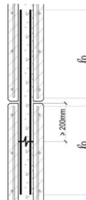
Figure 2 - Reprise de bétonnage dans le cas de MCI superposés
