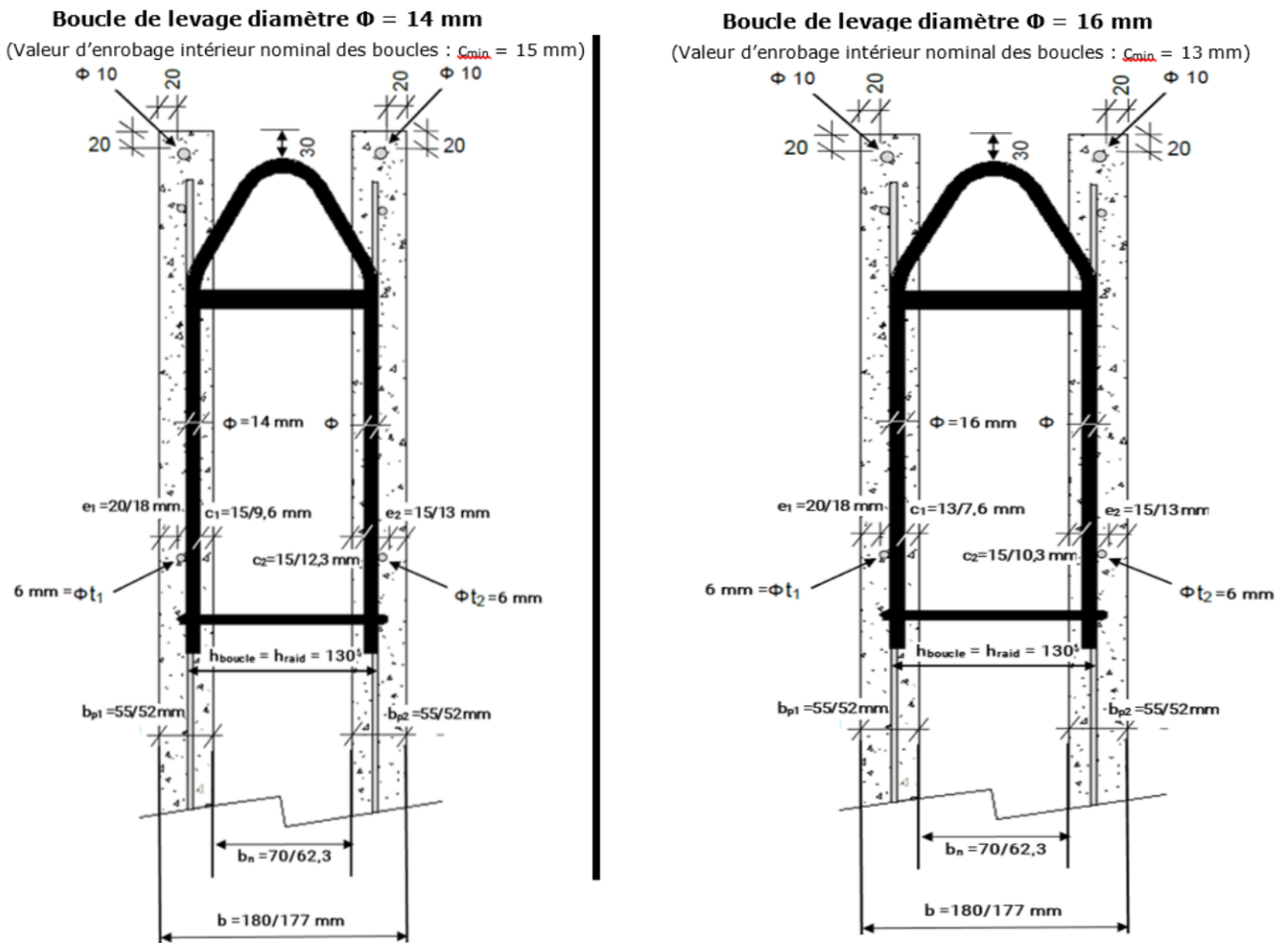
Figure 23 - COMPATIBILITE des BOUCLES de LEVAGE avec les PREMURS A2C – 18 cm
