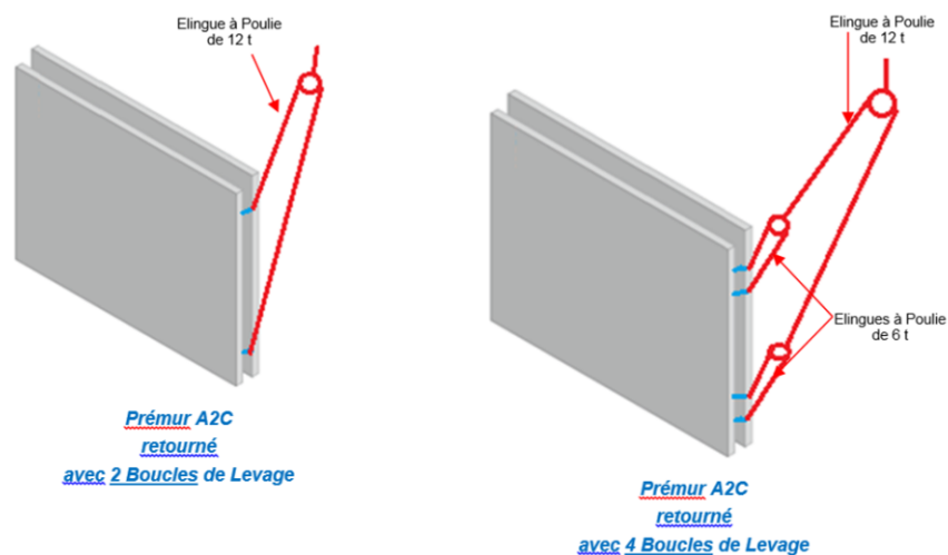
Figure 31 - MANUTENTION avec les BOUCLES de LEVAGE pour les Prémurs A2C à RETOURNER
