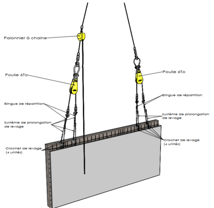
Figure 32 - MANUTENTION avec les INSERTS de LEVAGE Crochet A2C
