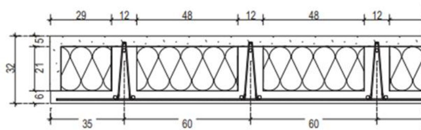
Figure 1 : Coupe du plancher dalle BB. Portées < 9,5m épaisseur dalle BB : 27 cm.
