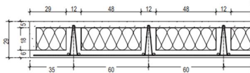
Figure 1 : Coupe du plancher dalle BB. Portées < 9m épaisseur dalle BB : 24 cm.
