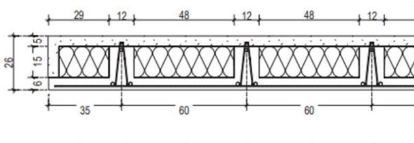
Figure 1 : Coupe du plancher dalle BB. Portées <8m50 épaisseur dalle BB : 21 cm.
