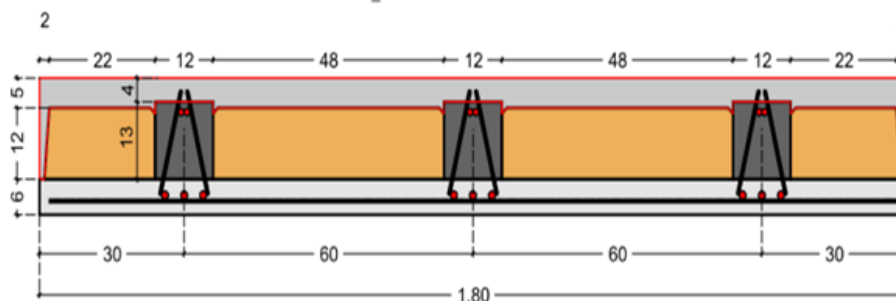
Figure 1 : Coupe du plancher dalle BB. Portées < 7m50 épaisseur dalle BB : 18 cm.
